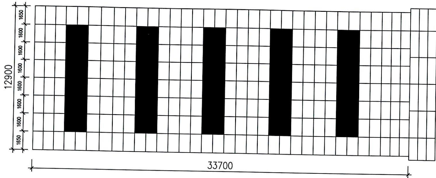
MẶT BẰNG MÁI SẴNH CHÍNH TẦNG 4
