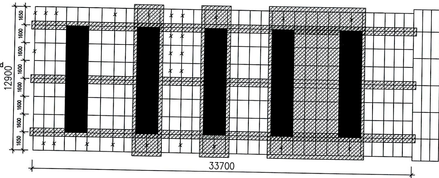
MẶT BẰNG MÁI SẴNH CHÍNH TẦNG 4 DÁN KEO CHỐNG THẤM
